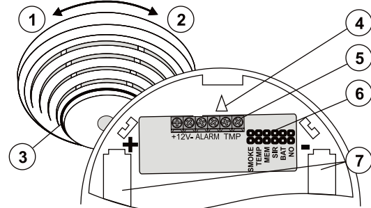
Abbildung 1 1 – Melder öffnen; 2 – Melder schließen; 3 – optische Statusanzeige; 4 – der Pfeil zeigt an, wo der Melder eingehängt werden soll; 5 – Klemmleiste; 6 – Drahtbrücken; 7 – Batteriefach
