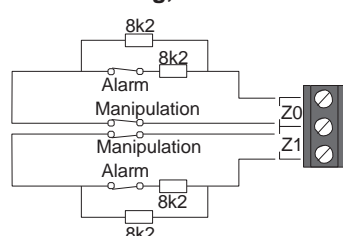
Abbildung 7 - Verdrahtungsarten
