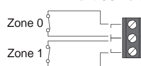
2-Draht CC-Verdrahtung
