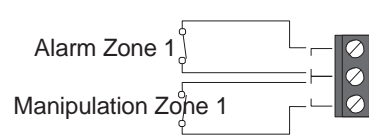
4-Draht CC-Verkabelung
