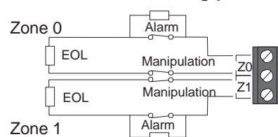
FSL-Verkabelung (Standard)
