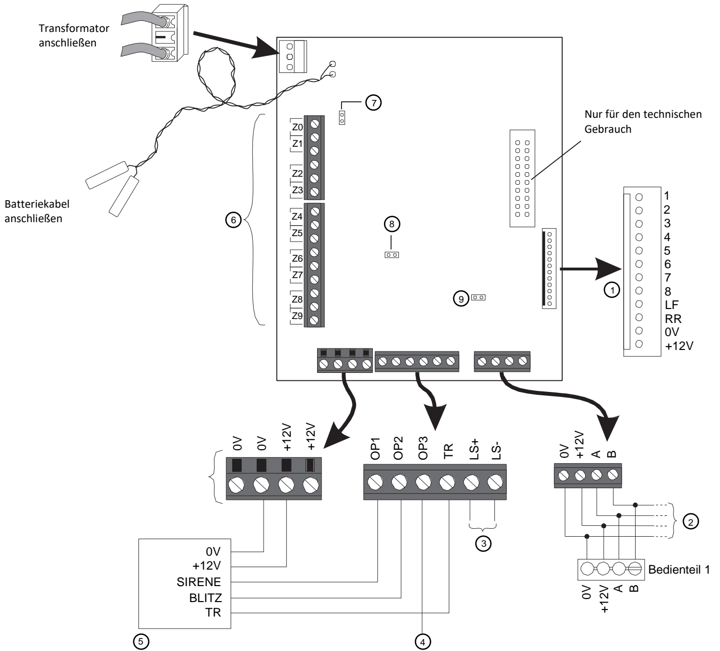
Abbildung 6 - Terxon SX PCB Übersicht
