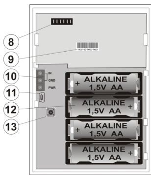
Abbildung 2: 8 – Anschluss für Kontrollsegmente; 9 – Produktionscode; 10 – Klemmen; 11 – miniUSB-Anschluss; 12 – Batterien; 13 – Sabotagekontakt
